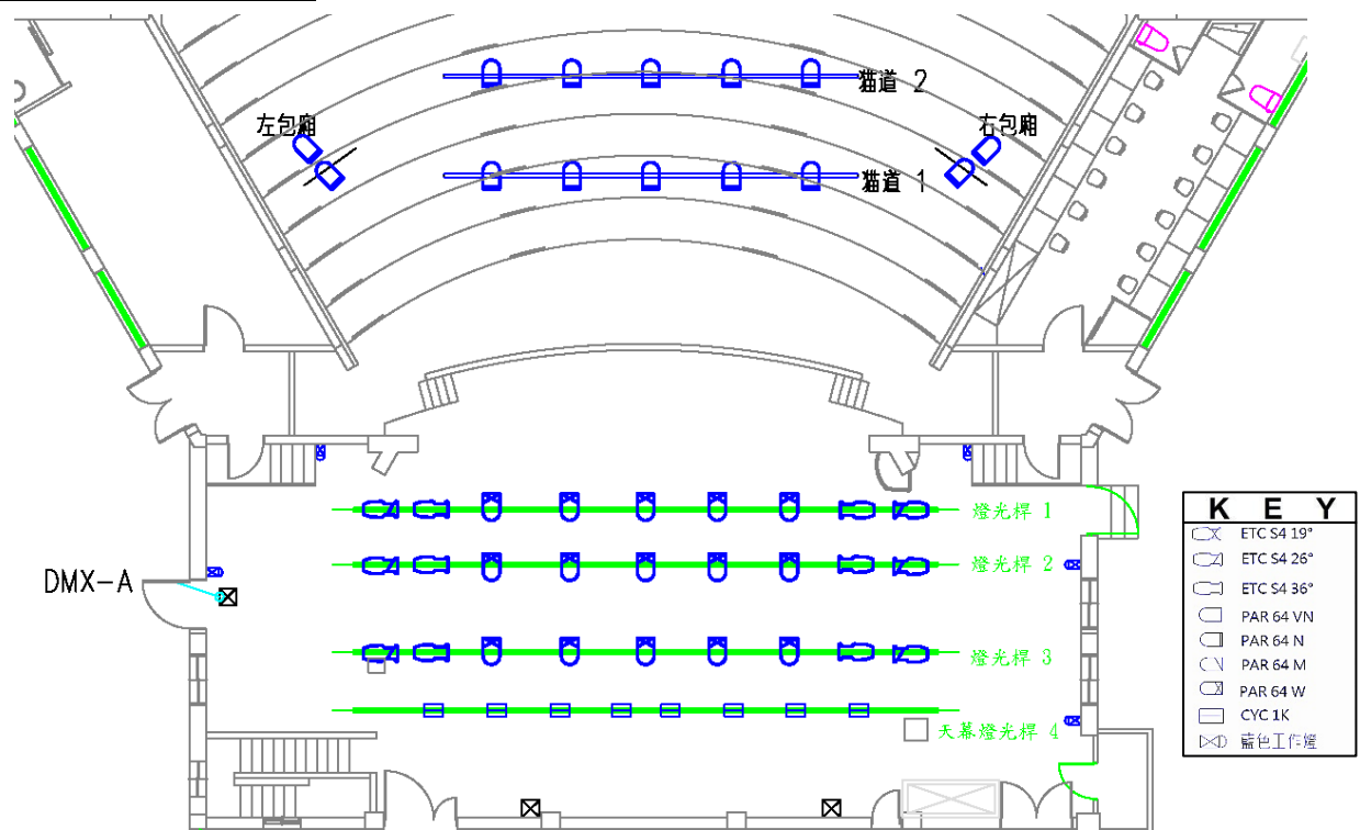
劇場燈光基本配置圖
