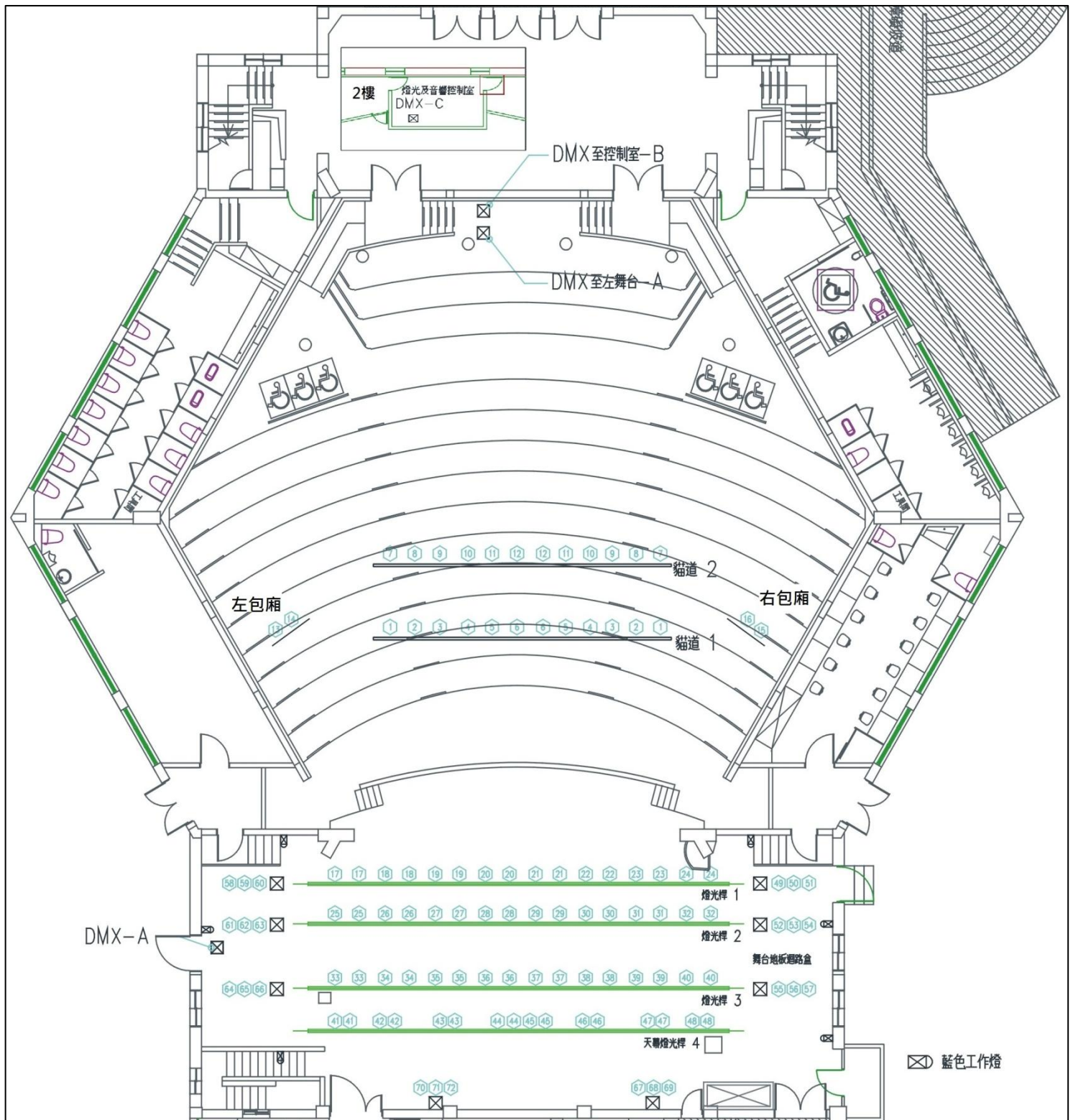
劇場燈光迴路圖
